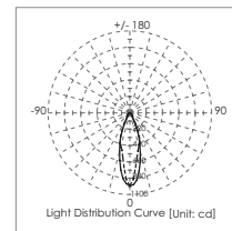
QR-CB51
