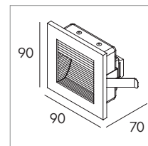
R6009S 3W
