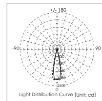
QR111
