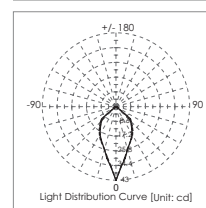
W6016H 1W
